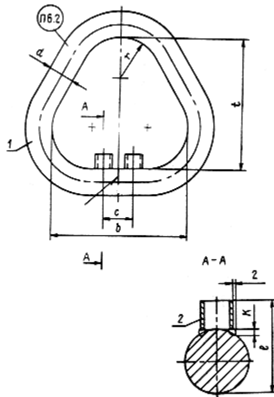
Рис. П.1.8. Звено типа Т, исполнение с двумя упорами:
