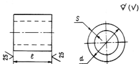
Рис. П.1.9. Упор типа У
