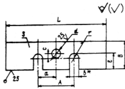
Рис. П.1.4. Ограничитель типа Ог
