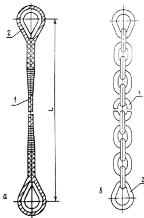
Рис. П.1.1.1. Канатная (а) и цепная (б) ветви стропа: а: 1 - канат, 2 - коуш; б: 1 - цепь, 2 - звено типа О
