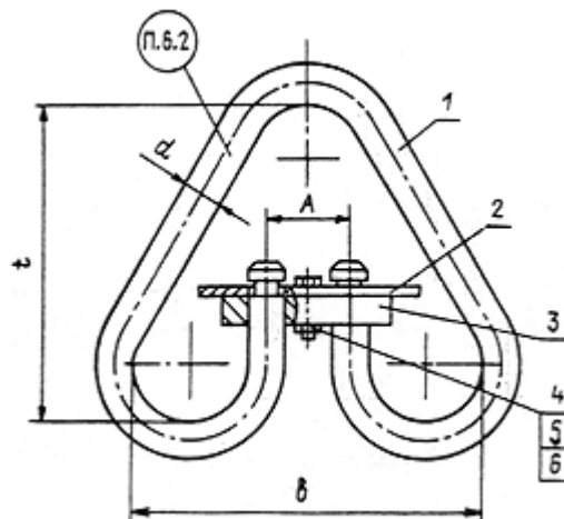
Рис. П.1.2. Звено типа Рт1: 1 - скоба, 2 - ограничитель, 3 - планка, 4 - болт по ГОСТ 7798, 5 - гайка по ГОСТ 5919, 6 - шплинг по ГОСТ 397
